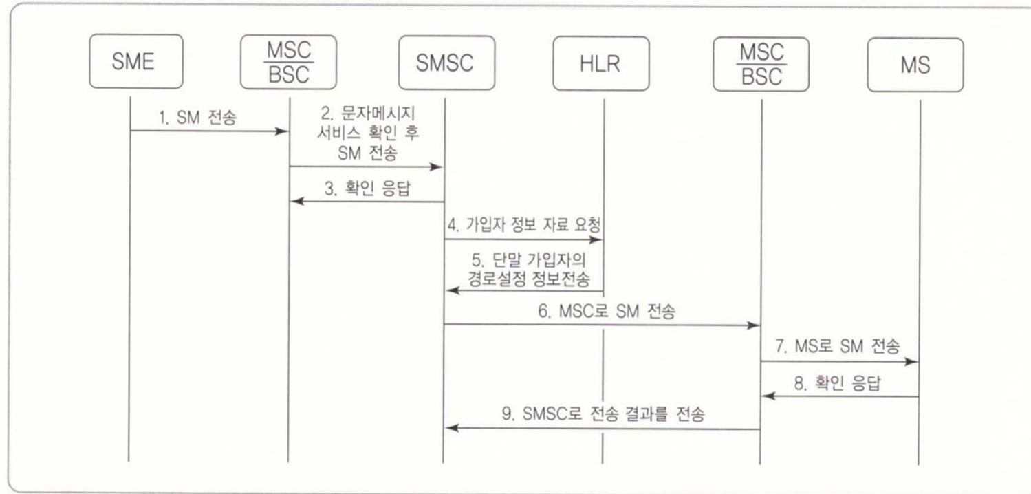
[그림 4-13] 단말기 메시지 전송 과정
